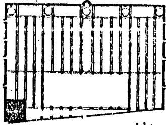
مخطط مسجد الكتبية MARRĀKŪŠ KUTŪBIYYA (VERS 1146 - VERS 1160)
